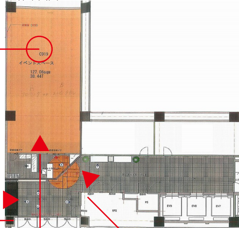
全体平面図
